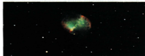
Así se pudo apreciar la Nebulosa Dumbell desde un telescopio instalado anoche en Ciudad Universitaria.
